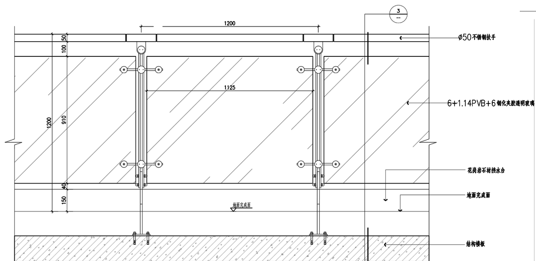
2 站厅下站台楼梯洞口挡水台及栏杆立面图 1:10
