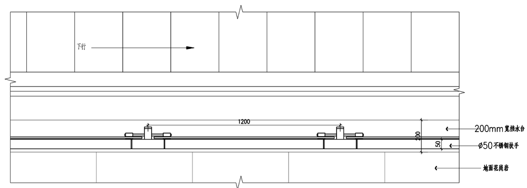
1 站厅下站台洞口挡水台及栏杆平面图 1:10
